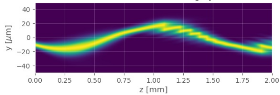
Normalizerad intensitet längs y-axeln
