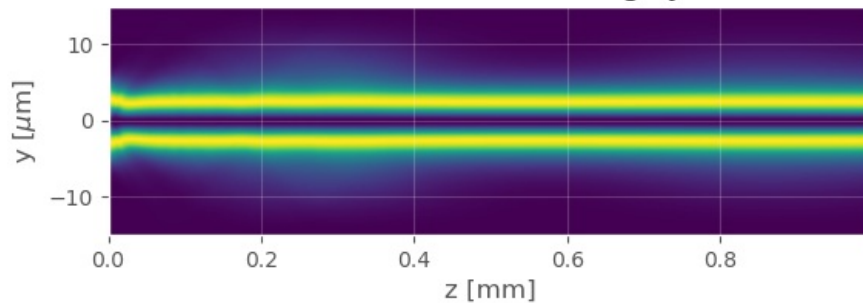
Normalizerad intensitet längs y-axeln
